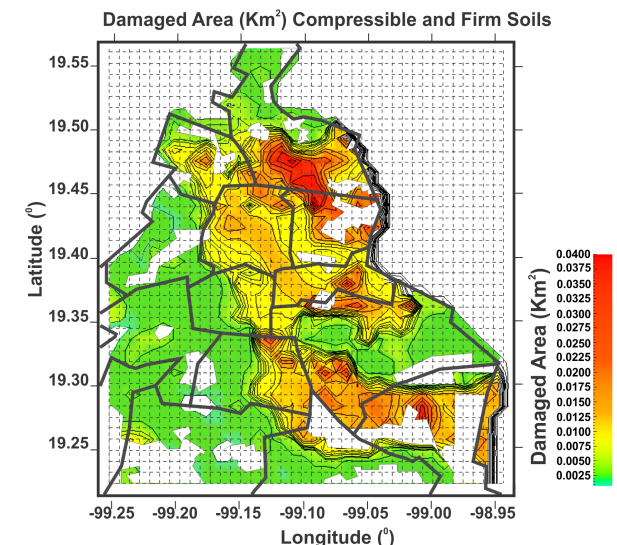
Estimación preliminar de los daños esperados por km 2 en construcciones habitacionales de uno a tres pisos en la Ciudad de México para un escenario sísmico de un evento de magnitud Mw 8.5 con epicentro en las costas del estado de Guerrero.
