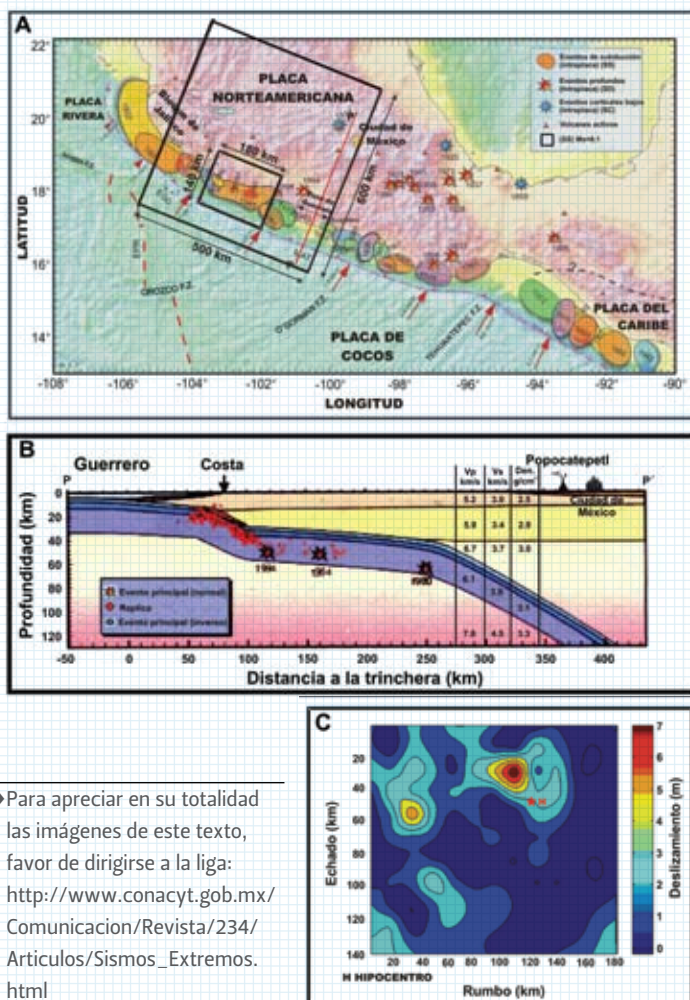
» FIGURA 1. A) Proyección en la superficie del volumen finito (500x600x124km 3 ) utilizado para el modelado del sismo extremo de Michoacán, México, del 19 de septiembre de 1985 Ms 8.1; B) Estructura geológica y parámetros geofísicos de las capas de la corteza terrestre del volumen finito; C) distribución de deslizamiento de la fuente sísmica correspondiente al sismo de 1985.
