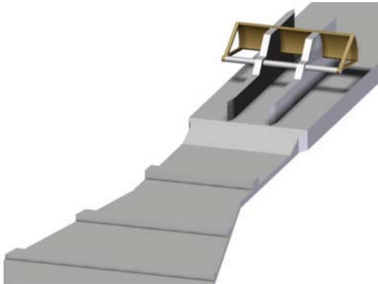
Figura 2. Simulación numérica de la estructura de control.
