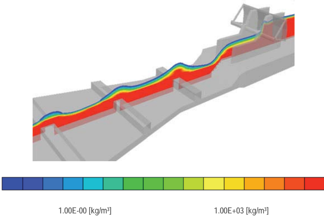
Figura 5. Contornos de densidad.
