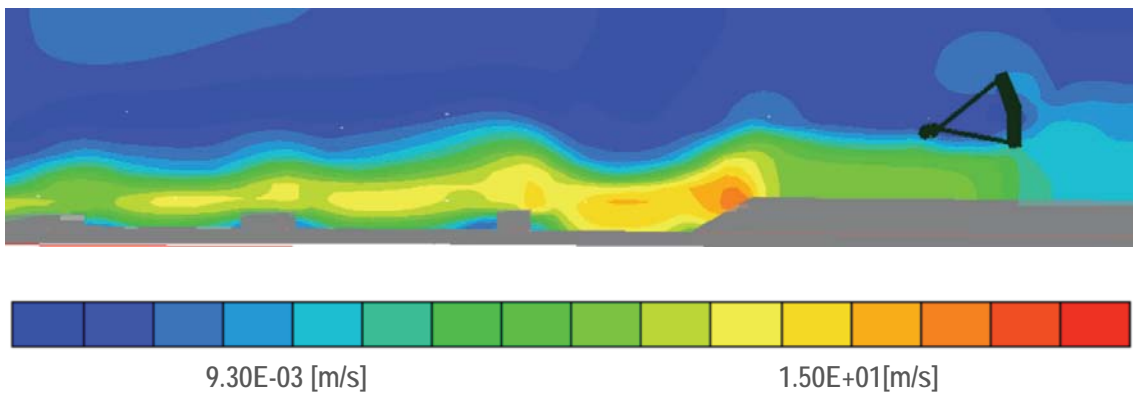
Figura 6. Contornos de velocidad.
