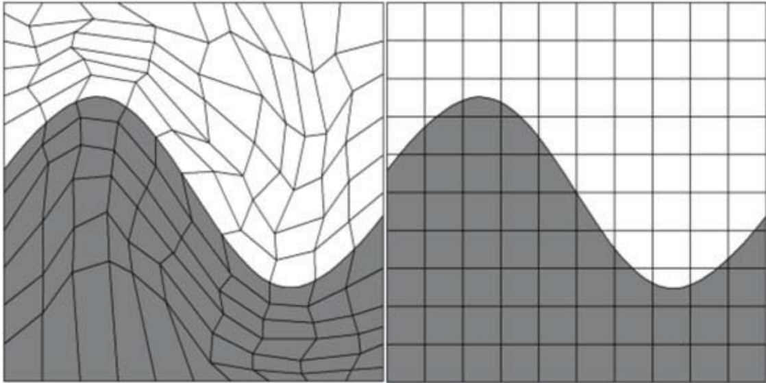
Figura 3. Métodos de estudio para el tratamiento de la superficie libre.
