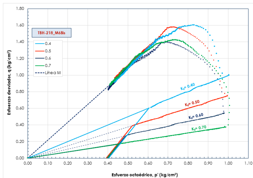
Curvas p' vs q para muestras del mismo horizonte, variando el valor de K_0 en la etapa de consolidación anisotrópica
