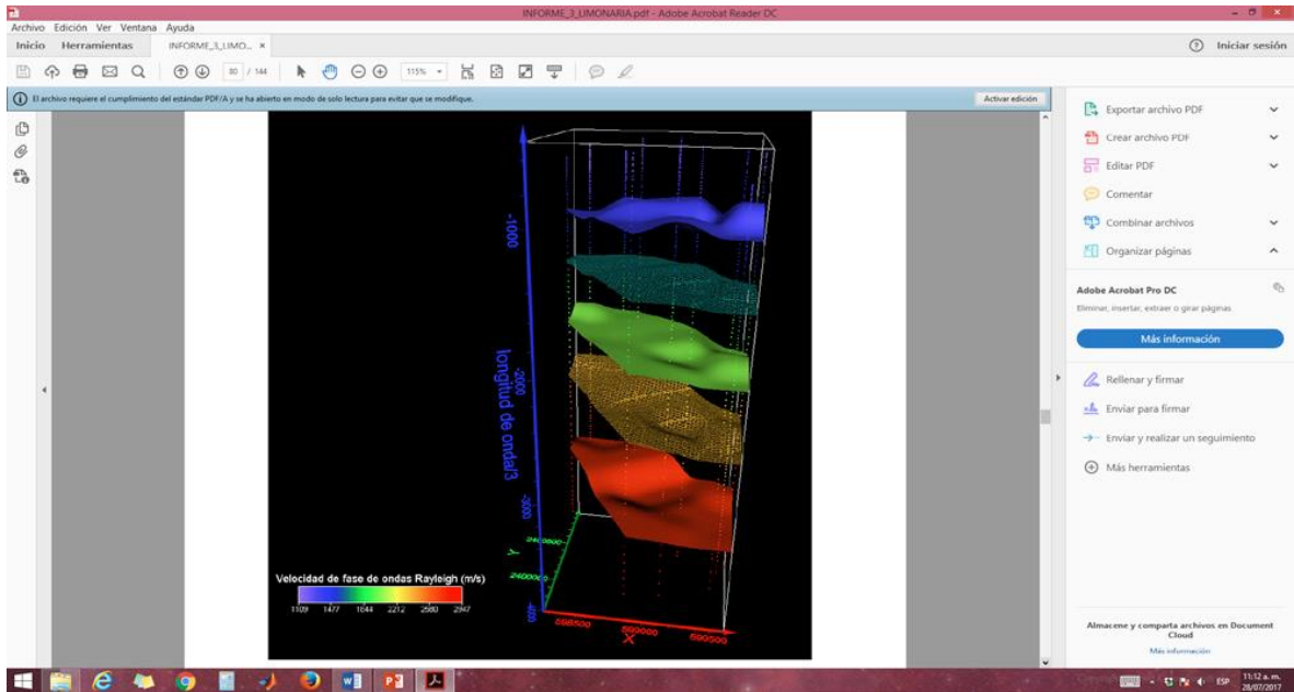
Figura 2. Modelo tridimensional obtenido a partir de las curvas de dispersión de velocidades de fase de las ondas de Rayleigh
