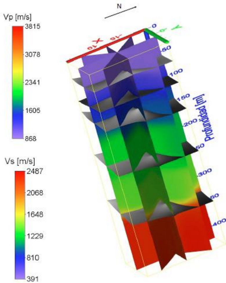
Figura 1. Distribución del arreglo de estaciones en el Jardín Botánico de la BUAP (arriba a la izquierda). Curva de dispersión obtenida (arriba a la derecha). Modelo tridimensional de la estructura de velocidades estimada (abajo)
